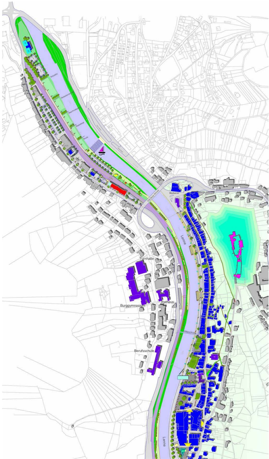
Städtebauliches Konzept - Gesamtplan
